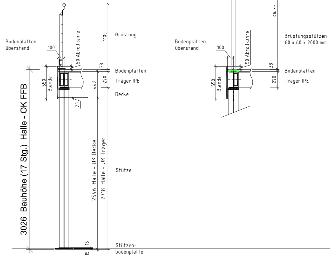
SCHNITT HEA-Stütze 17 Stg. Brüstung PRIMO 110 Blende - Decke
